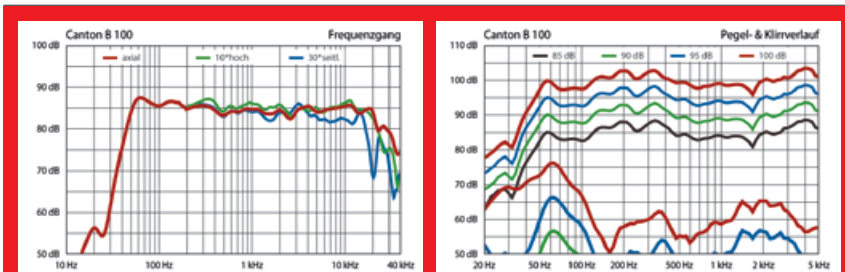
Canton hat die B100 linear abgestimmt, im gesamten Übertragungsbereich zeigen sich nur minimale Welligkeiten. Die Abstrahlung in den Raum gelingt sehr homogen, wie die kaum auseinanderdriftenden Frequenzgänge belegen. Der Bass reicht hinab bis 40 Hz, der Maximalpegel wird erst bei 106 dBspl erreicht. Die Canton ist ein unkritisch zu befeuernder Lautsprecher mit der AUDIO-Kennzahl 61 .
